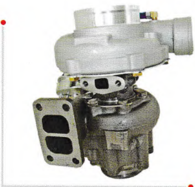
名称：涡轮增压器 Name : Turbocharger 型号：TBP4 Model : TBP4 主机厂号：1118010S-BKZ OEM : 1118010S-BKZ 应用发动机：锡柴 Type : Stannic bavin
