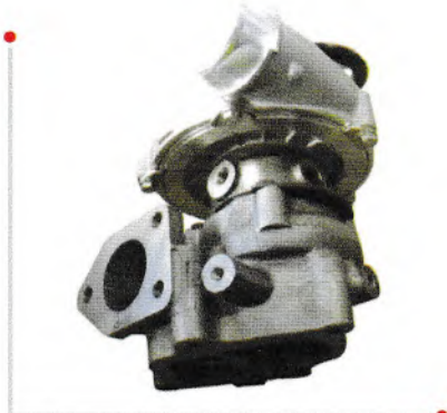
名称：涡轮增压器 Name : Turbocharger 型号：GT17 Model : GT17 主机厂号：28200 4A001 OEM : 28200 4A001
