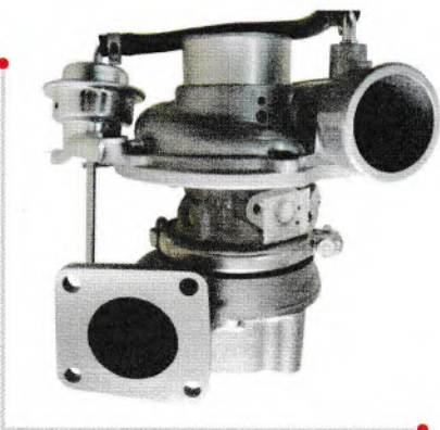
名称：涡轮增压器 Name : Turbocharger 型号：RHF5 Model : RHF5 主机厂号：1118010-850 OEM : 1118010-850 应用发动机：4KH1-TC Type : 4KH1-TC
