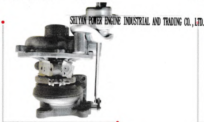
名称：涡轮增压器 Name : Turbocharger 型号：RHB5 Model : RHB5 主机厂号：897160801 OEM : 897160801 应用发动机：4JB1 Type : 4JB1
