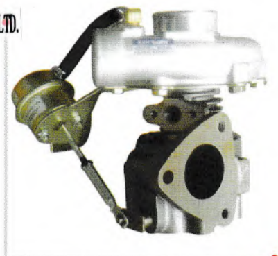
名称：涡轮增压器 Name : Turbocharger 型号：GT22 Model : GT22 主机厂号：1118300SD OEM : 1118300SD 应用发动机：江铃 Type : JMC
