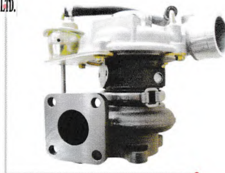
名称：涡轮增压器 Name : Turbocharger 型号：RHF4 Model : RHF4 主机厂号：XNZ11186000 OEM : XNZ11186000 应用发动机：4JB1 Type : 4JB1
