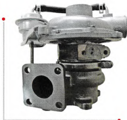
名称：涡轮增压器 Name : Turbocharger 型号：RHF4 Model : RHF4 主机厂号：1118010-44 OEM : 1118010-44 应用发动机：4JB1-TCT Type : 4JB1-TCT
