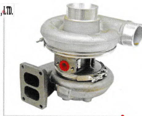
名称：涡轮增压器 型号：4LGK 应用发动机：奔驰
