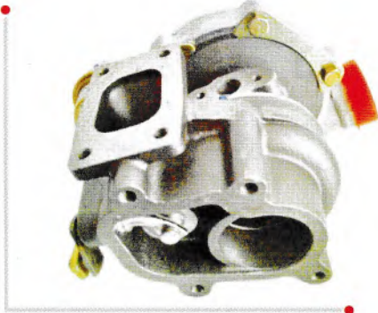
名称：涡轮增压器 Name : Turbocharger 型号：GT22 Model : GT22 主机厂号：1118010G5X4 OEM : 1118010G5X4 应用发动机：大柴498 Type : 大柴498
