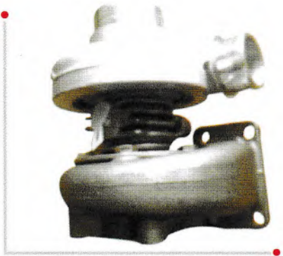
名称：涡轮增压器 Name : Turbocharger 型号：GT22 Model : GT22 应用发动机：福田483 Type : Foton 483
