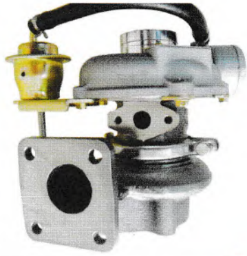
名称：涡轮增压器 Name : Turbocharger 型号：RHF4 Model : RHF4 主机厂号：97300198 OEM : 97300198 应用发动机：SOFIM8140.43 Type : SOFIM8140.43
