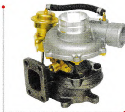
名称：涡轮增压器 Name : Turbocharger 型号：RHB5 Model : RHB5 主机厂号：97210034 OEM : 97210034 应用发动机：索菲姆8140.47 Type : Sofim 8140.47
