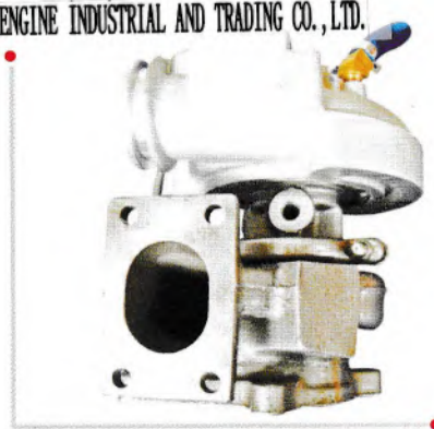
名称：涡轮增压器 Name：Turbocharger 型号：HE221W Model：HE221W 主机厂号：4047105 OEM：4047105 应用发动机：ISDe4 Type：ISDe4
