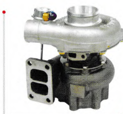
名称：涡轮增压器 型号：TBP4 主机厂号：2674A059 应用发动机：帕金斯 Name : Turbocharger Model : TBP4 OEM : 2674A059 Type : PARKINS
