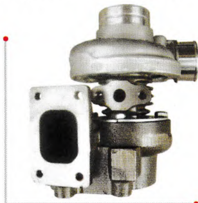
名称：涡轮增压器 型号：GT22 应用发动机：玉柴2115
